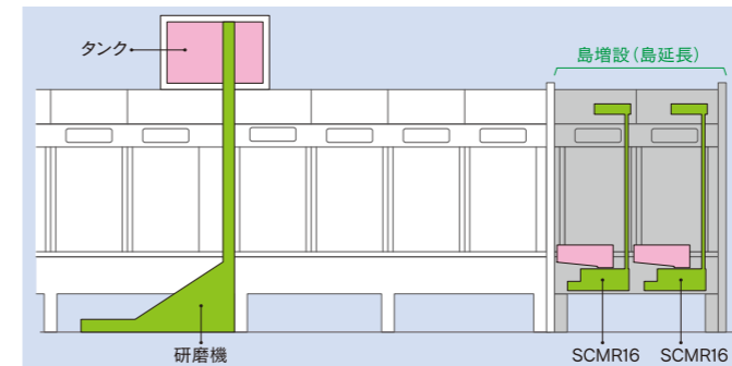
単体島システム「Isoletta(イゾレッタ)」
