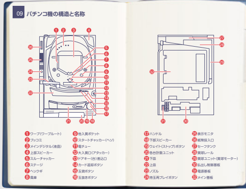
[遊技機の仕組みと名称]
