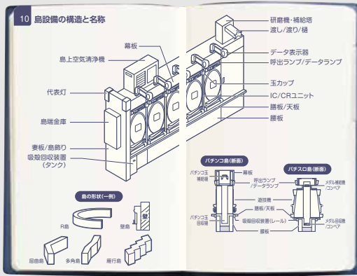
[島設備の構造と名称]
